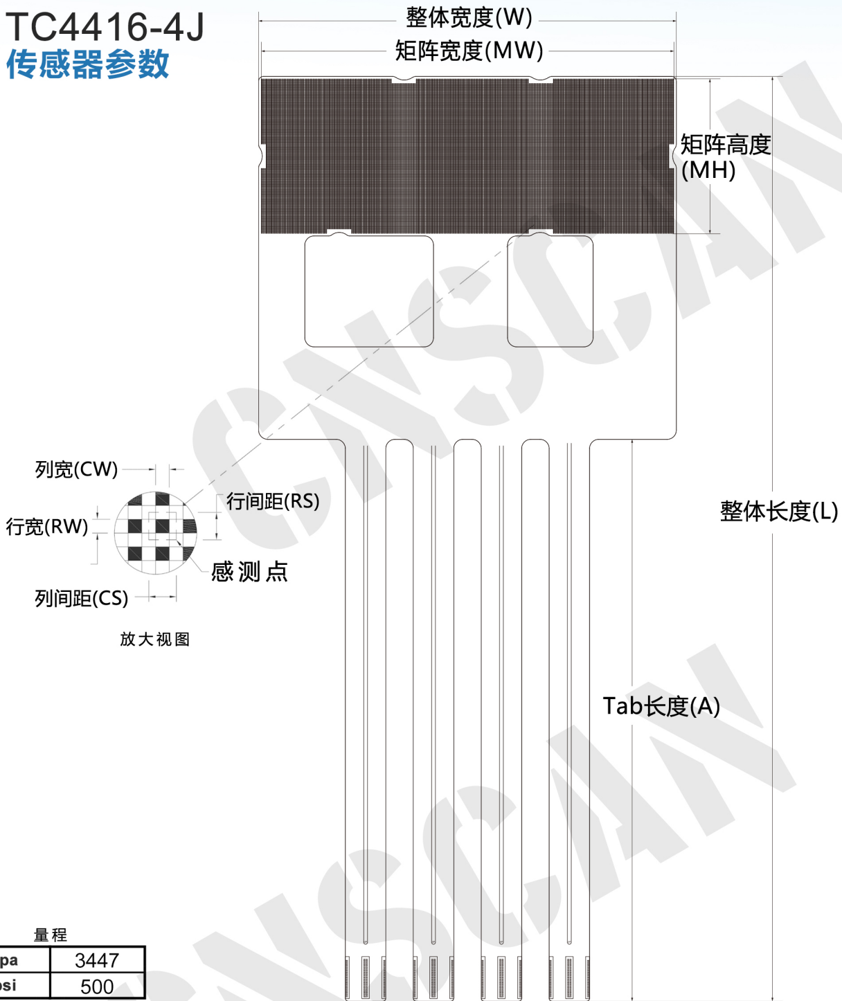
外形尺寸
