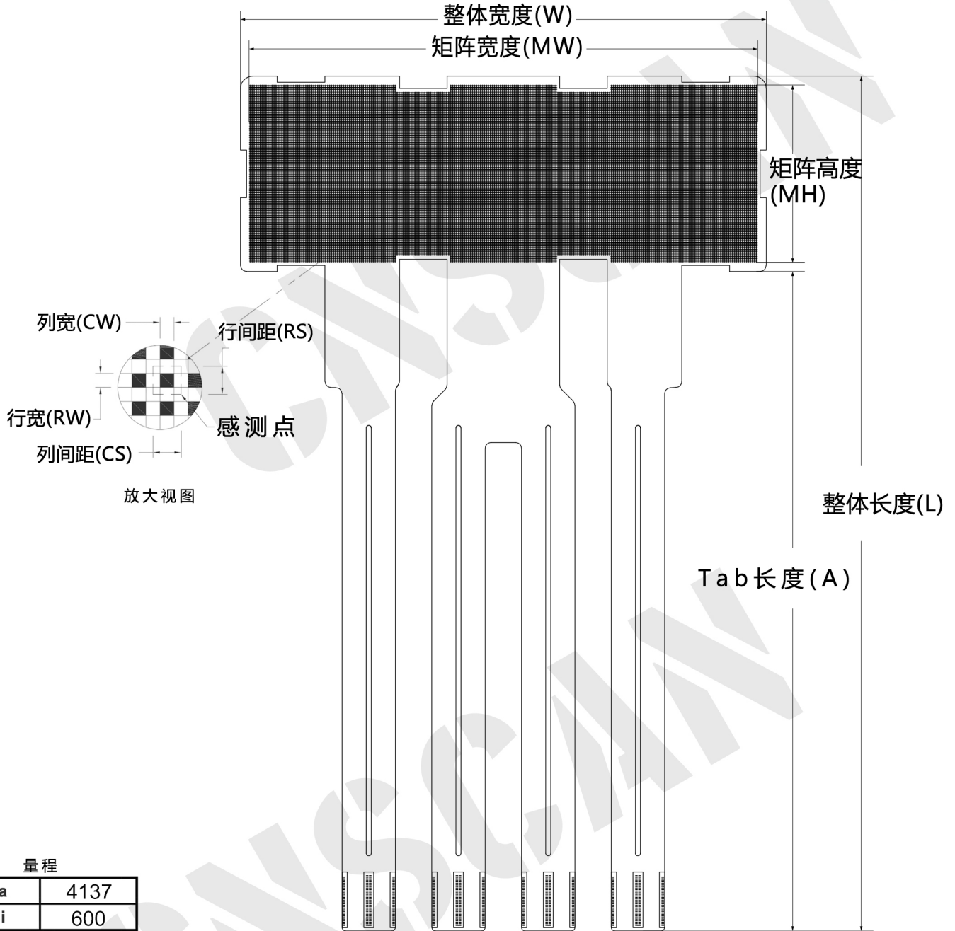
外形尺寸
