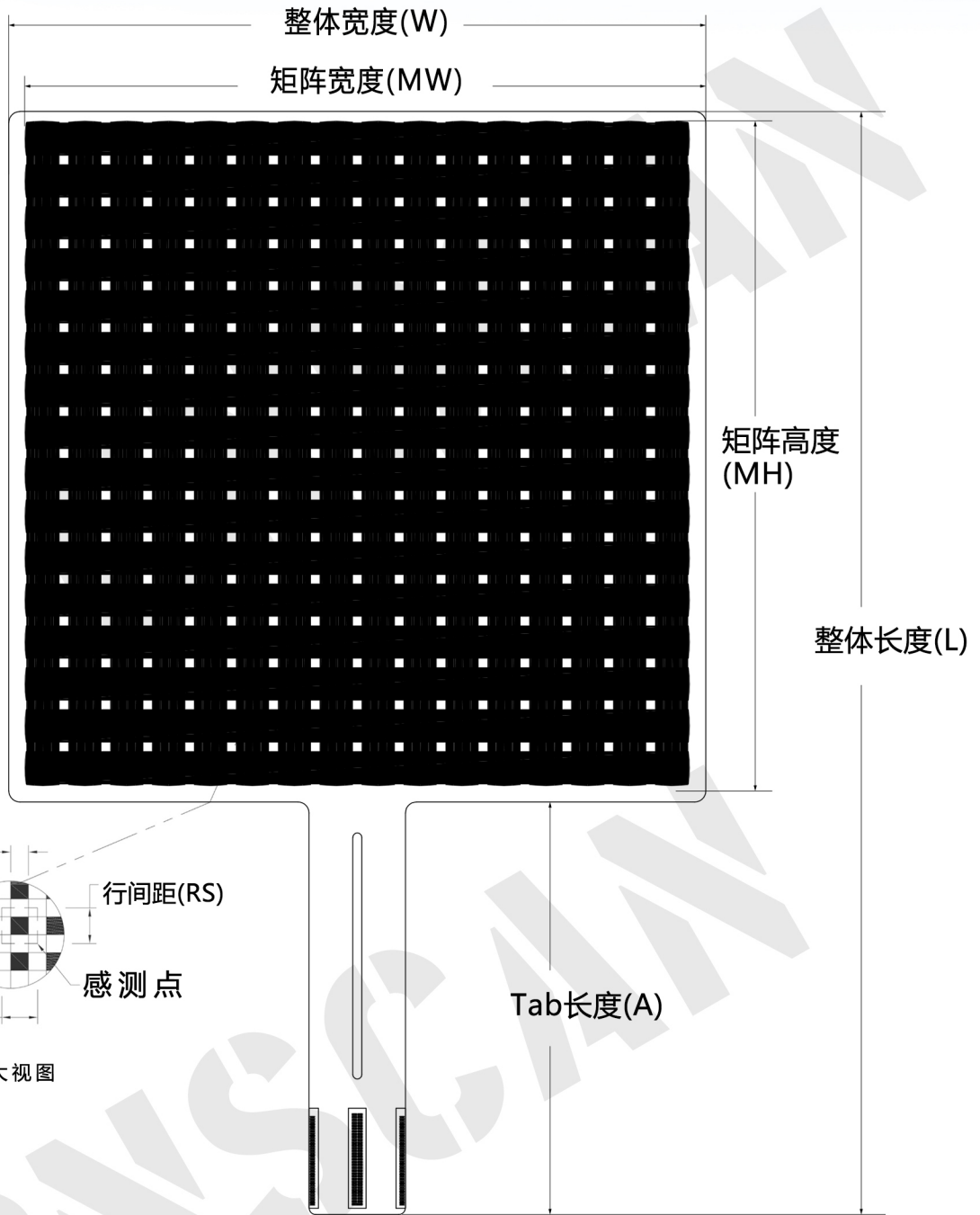
外形尺寸
