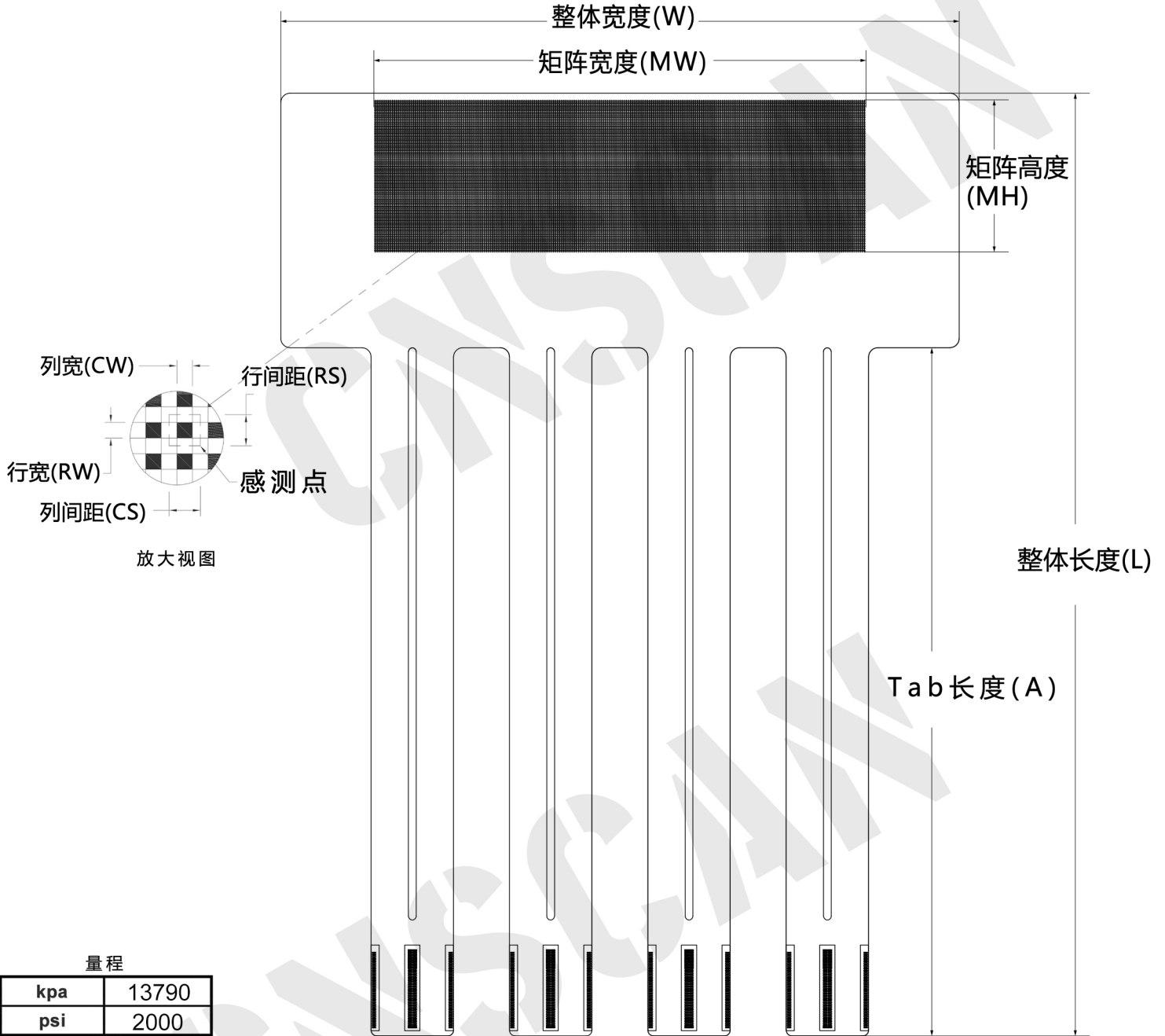
外形尺寸
