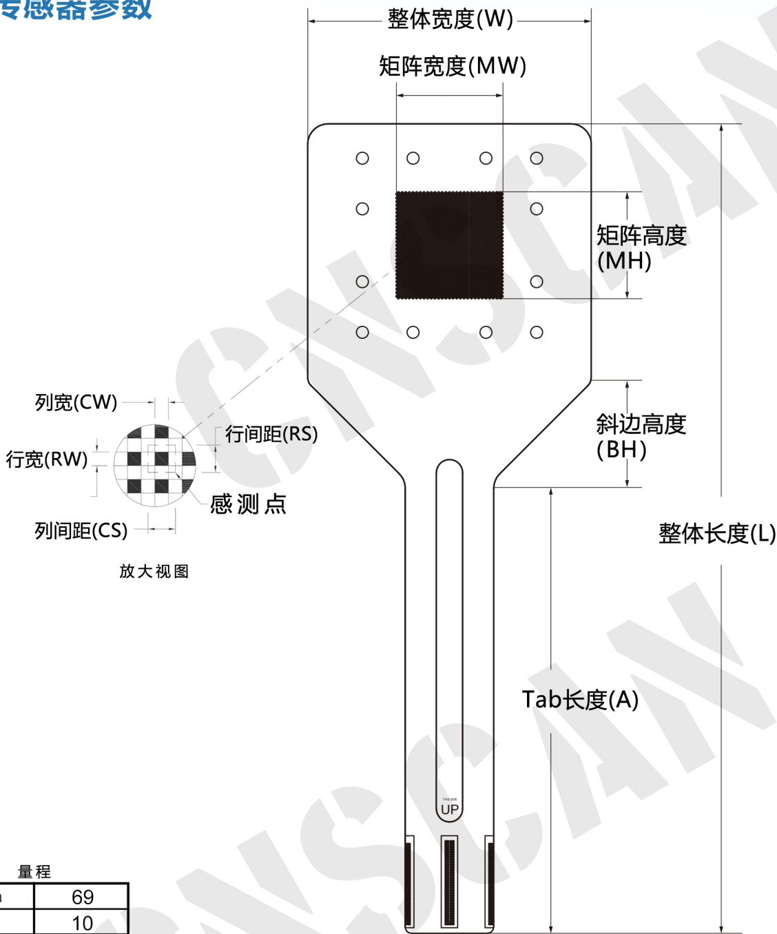
外形尺寸
