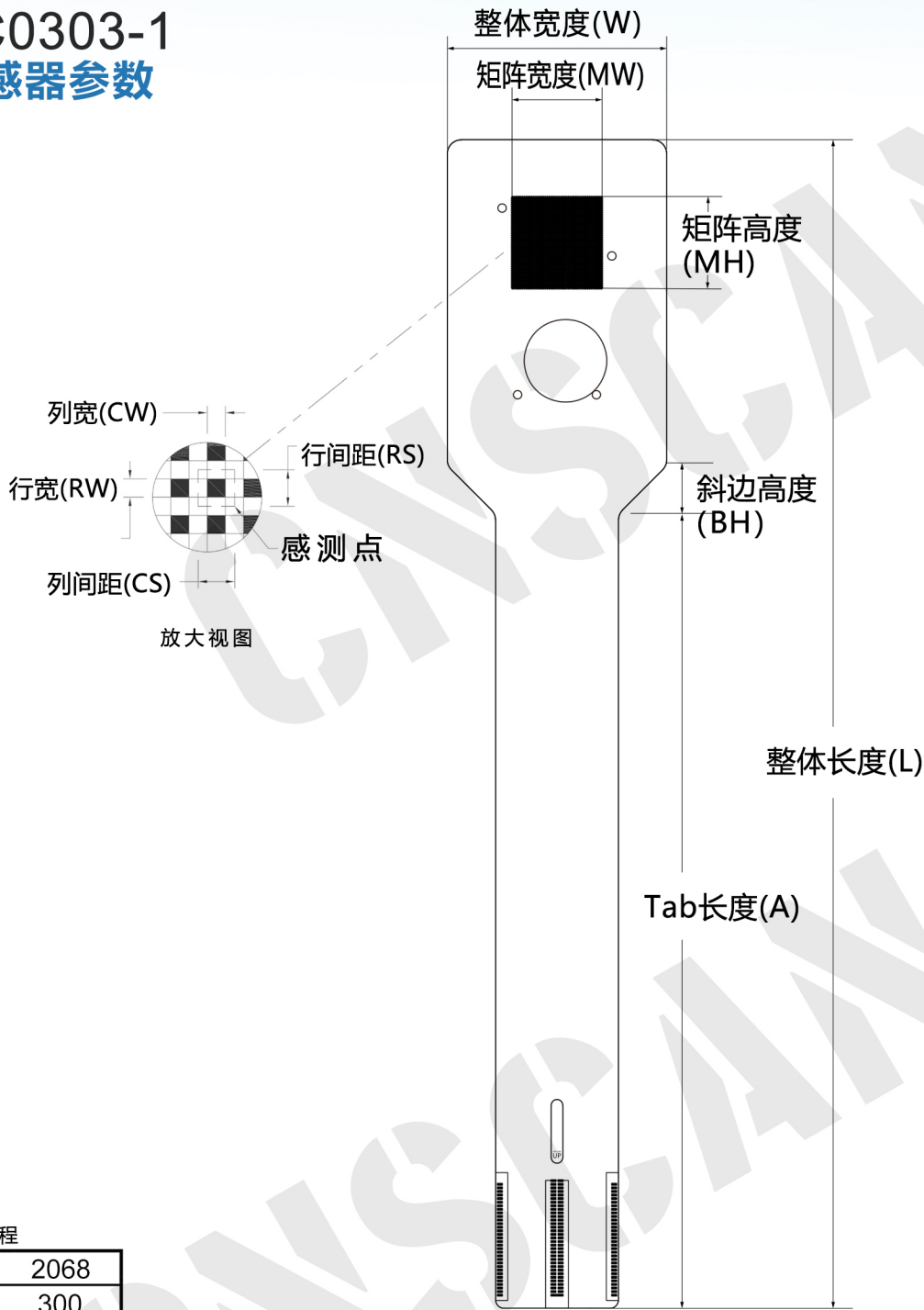
外形尺寸
