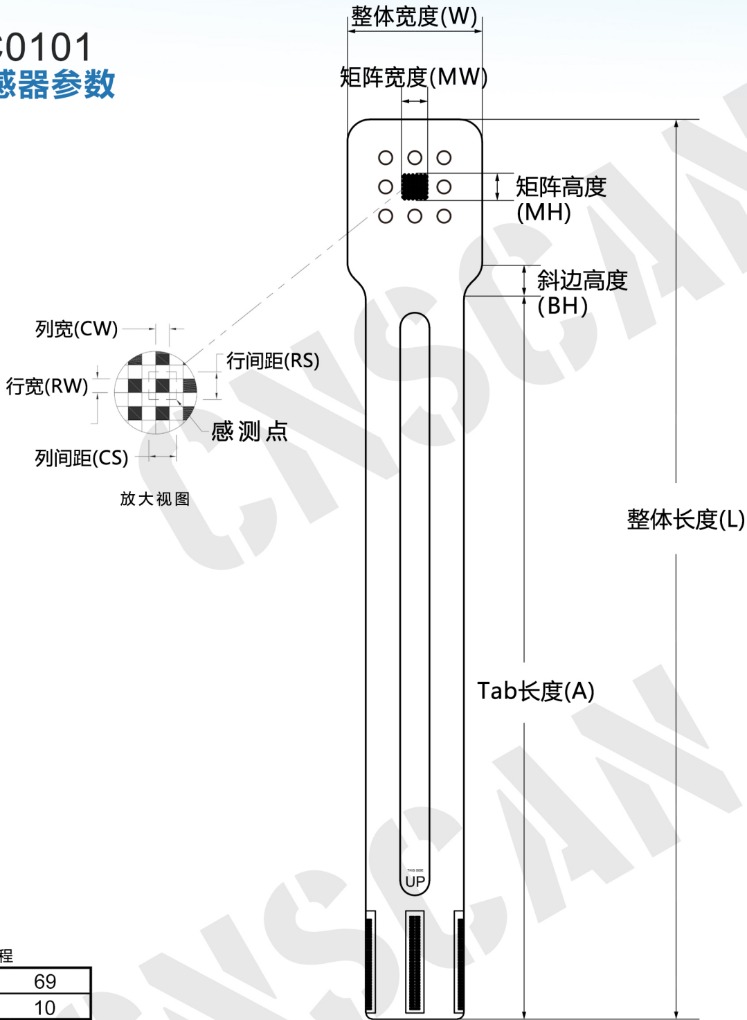
外形尺寸
