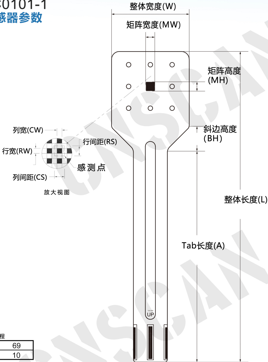
外形尺寸
