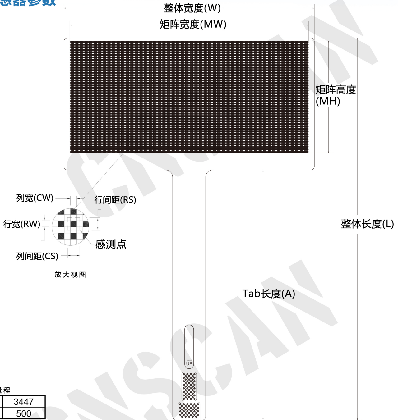
外形尺寸
