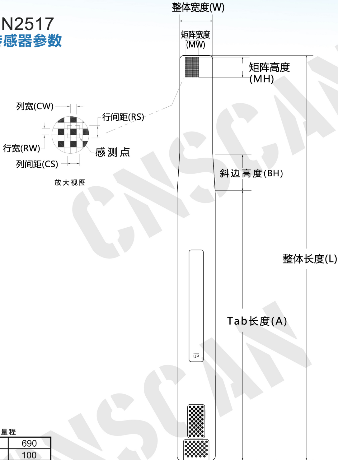
外形尺寸
