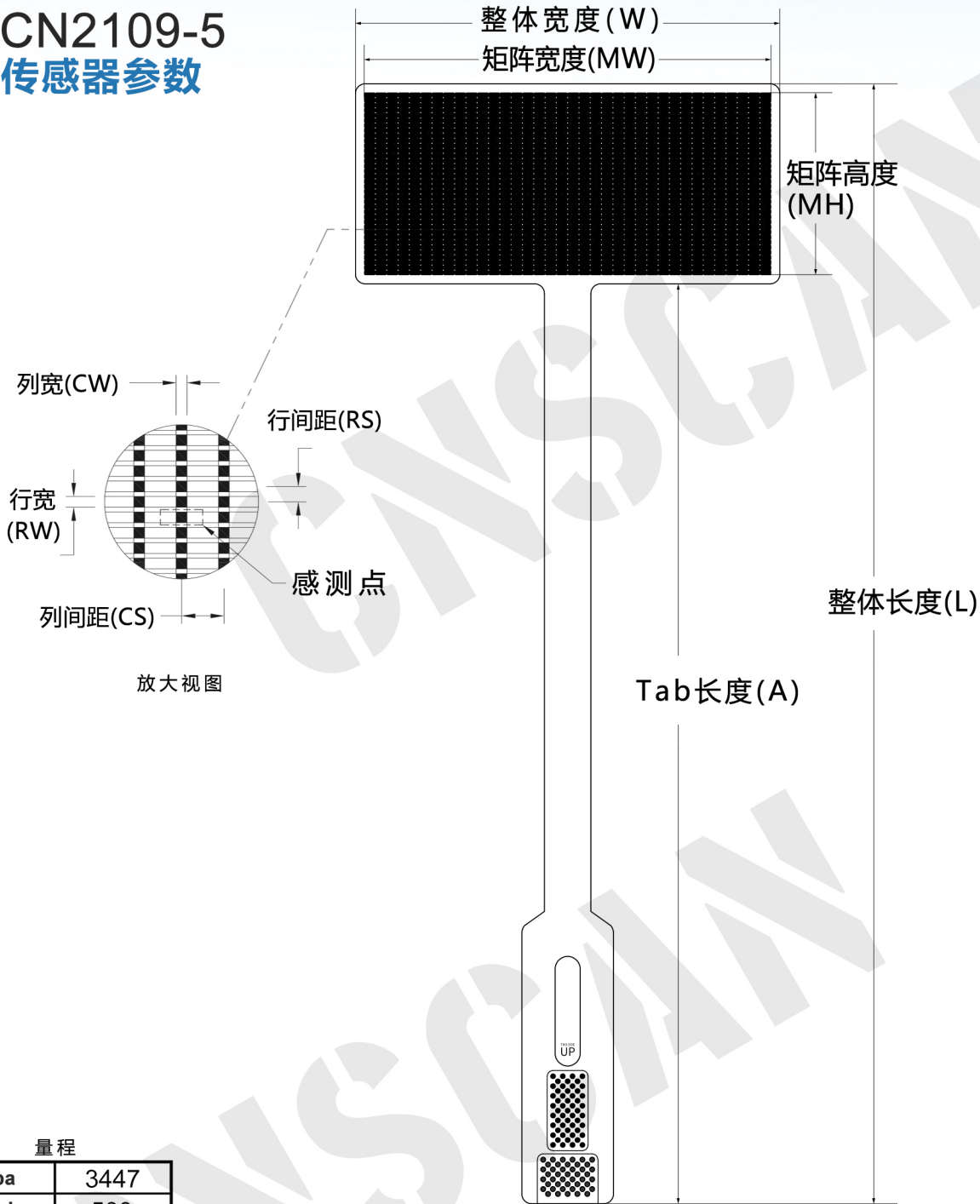
外形尺寸
