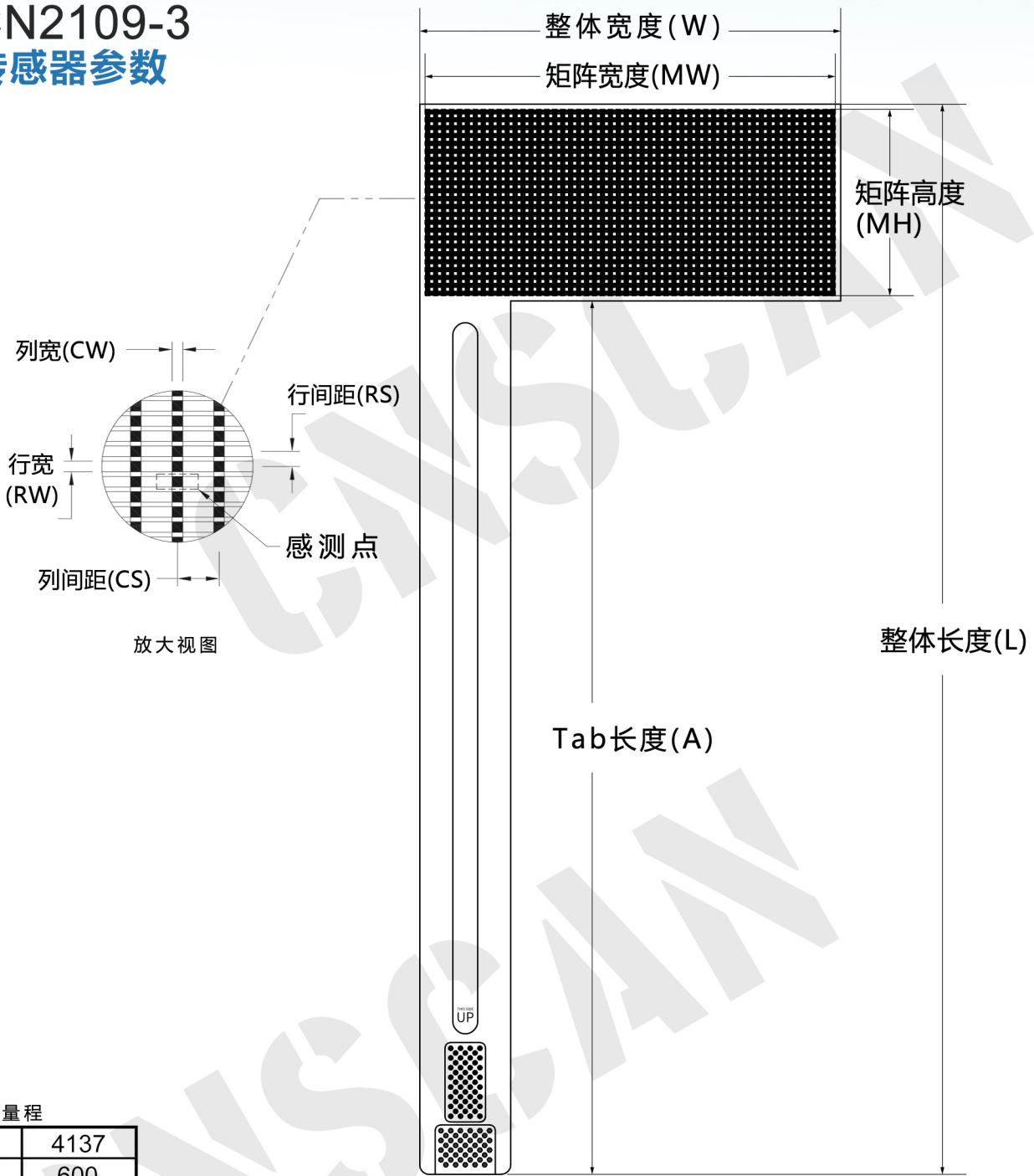
外形尺寸
