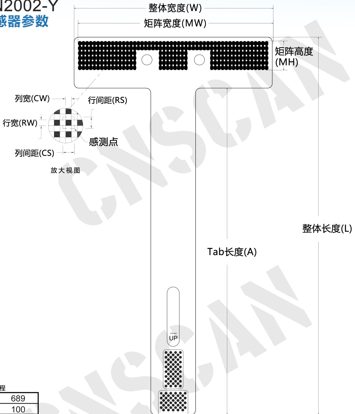
外形尺寸
