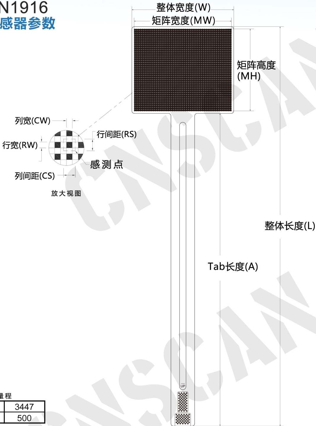
外形尺寸
