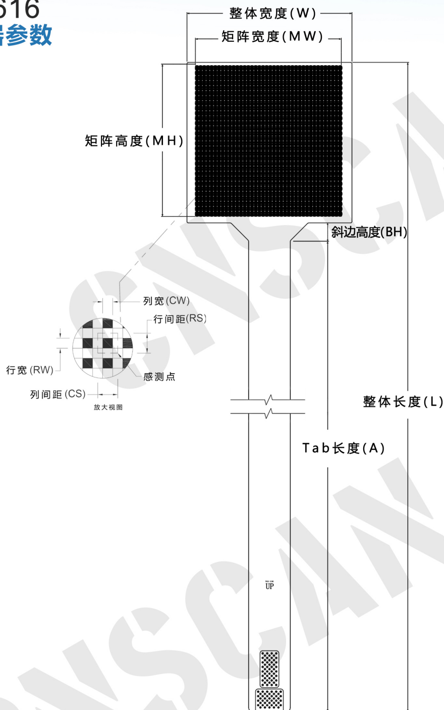
外形尺寸
