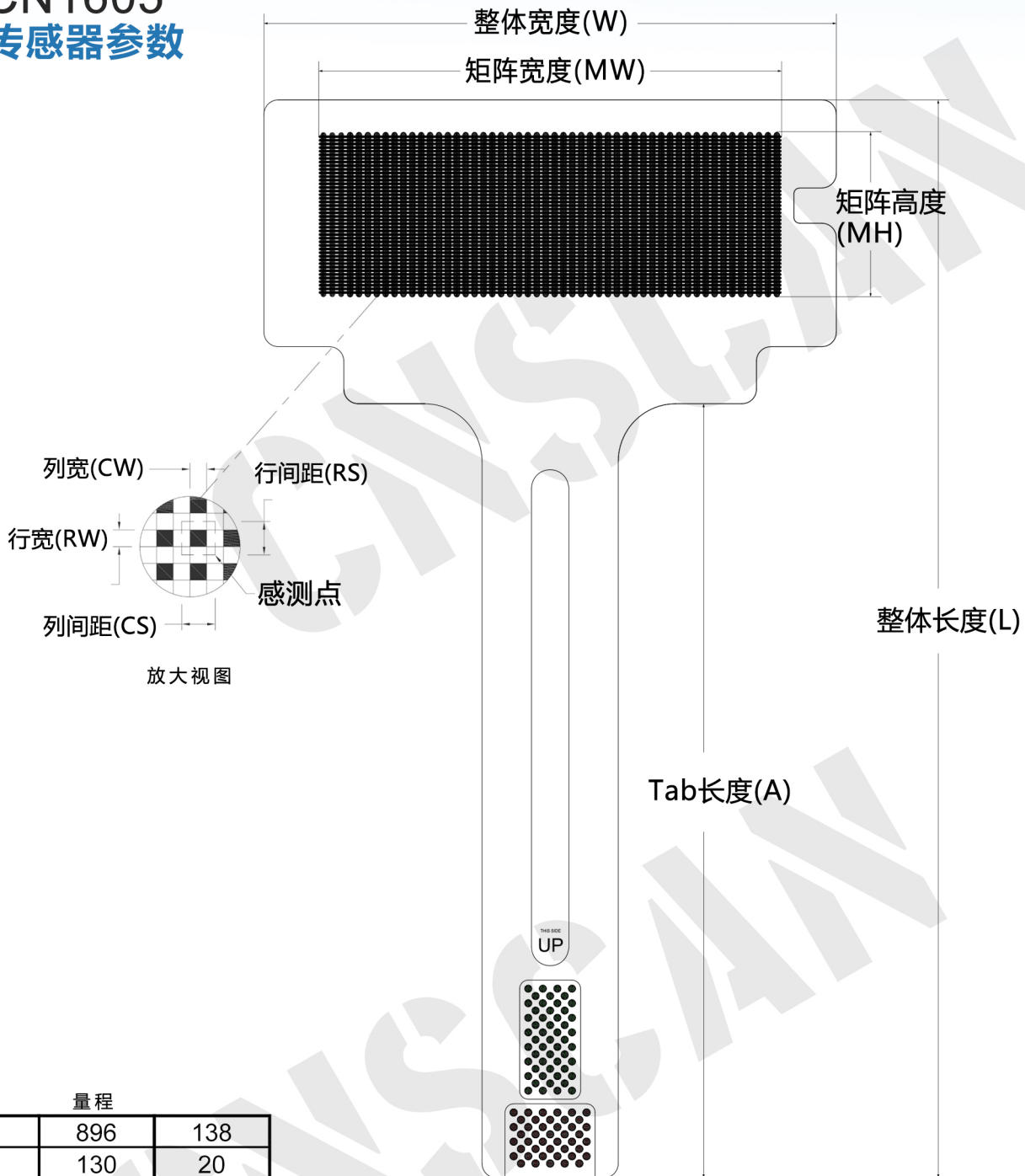
外形尺寸
