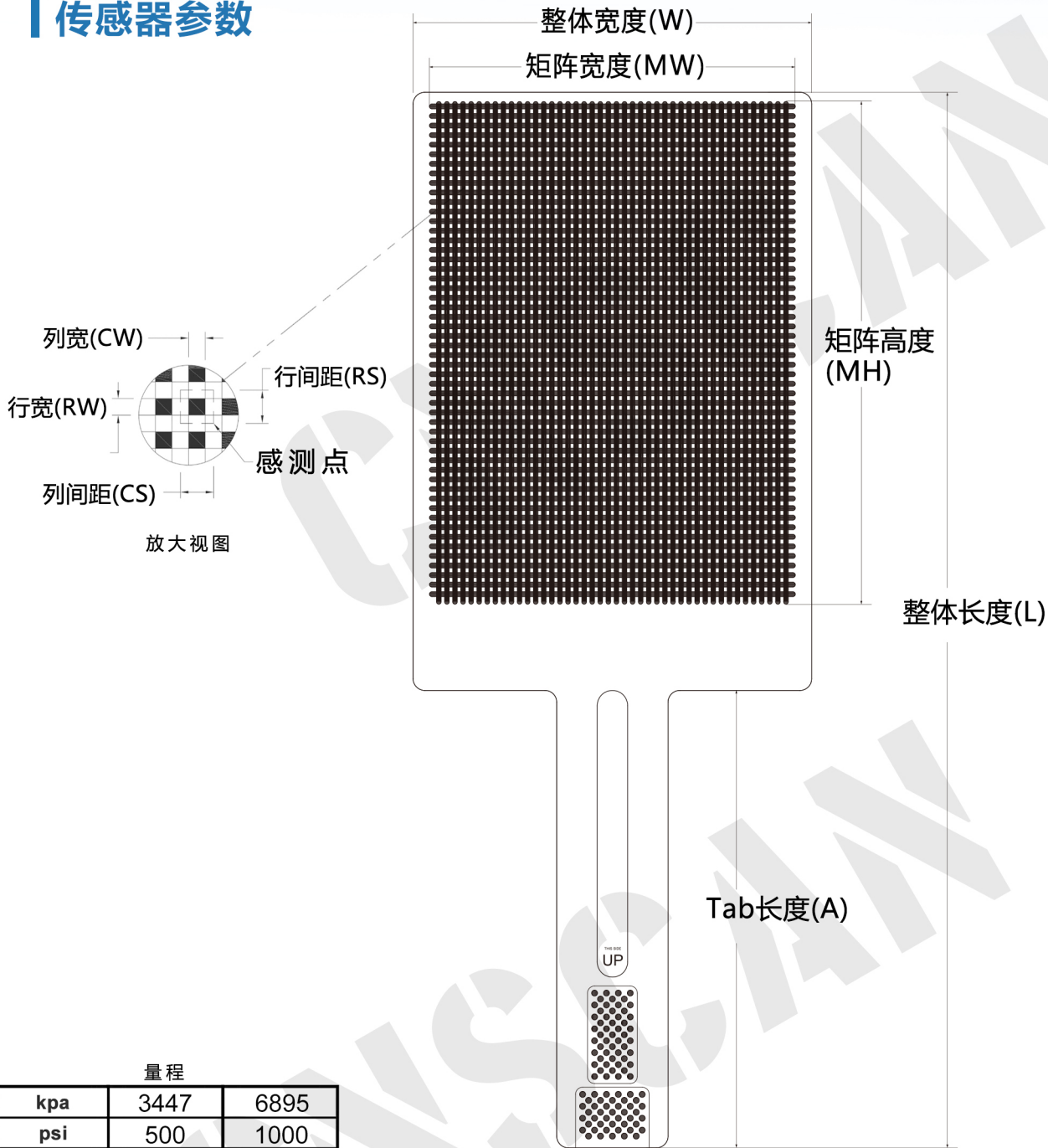
外形尺寸
