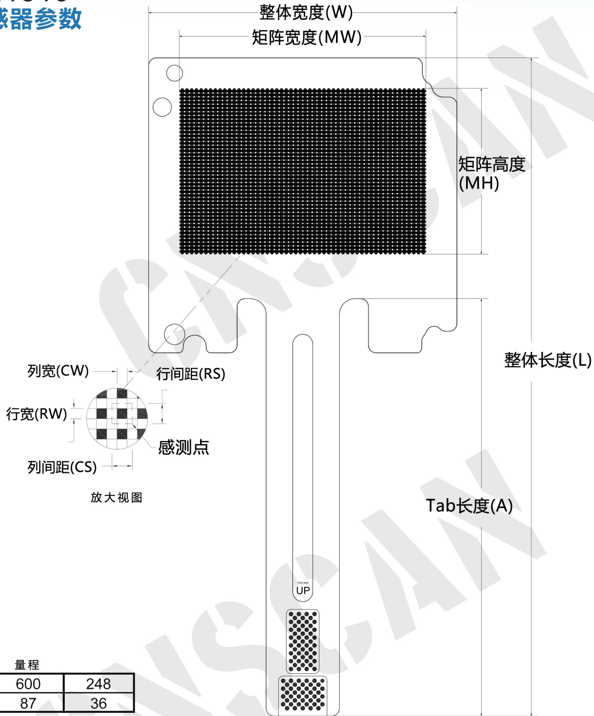
外形尺寸
