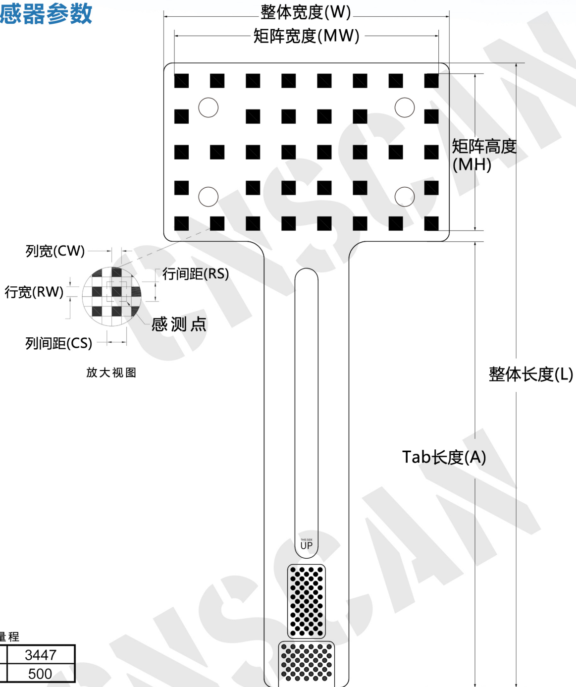
外形尺寸
