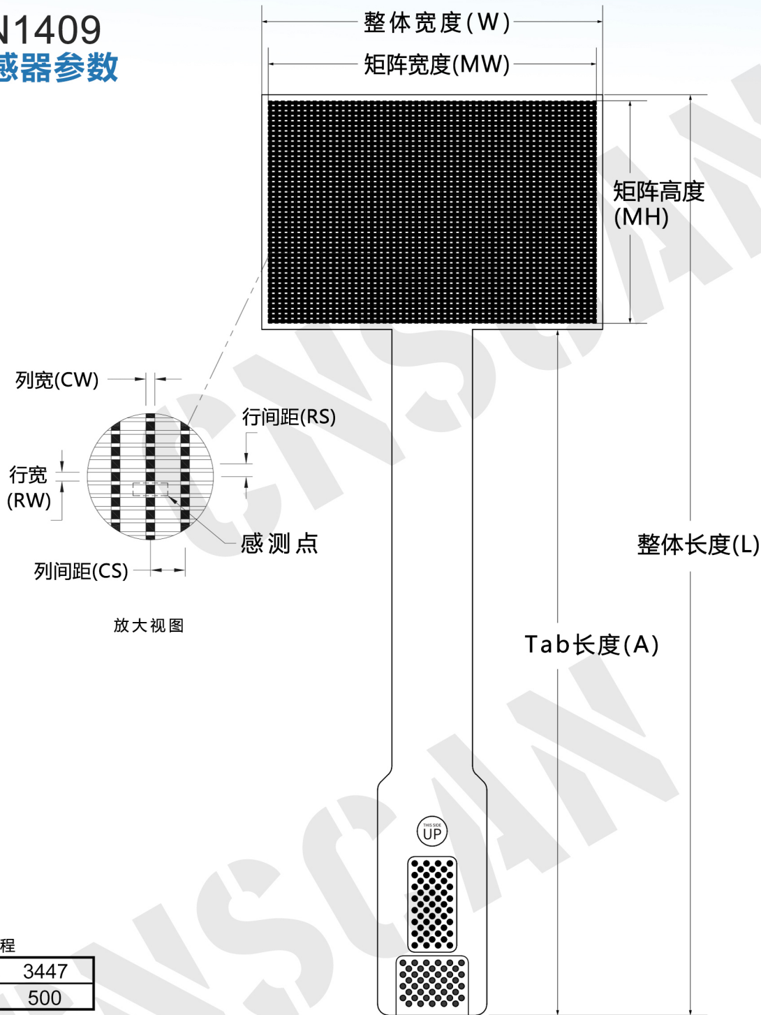
外形尺寸
