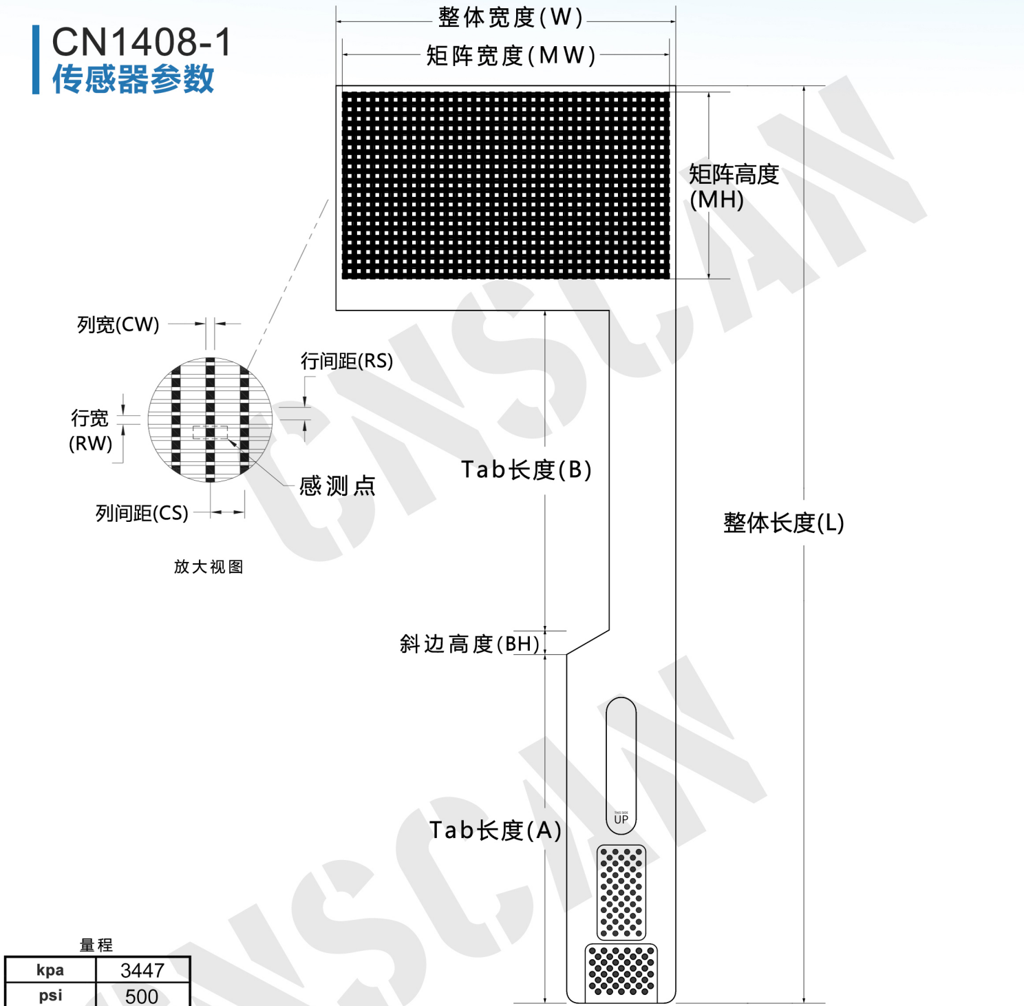
外形尺寸
