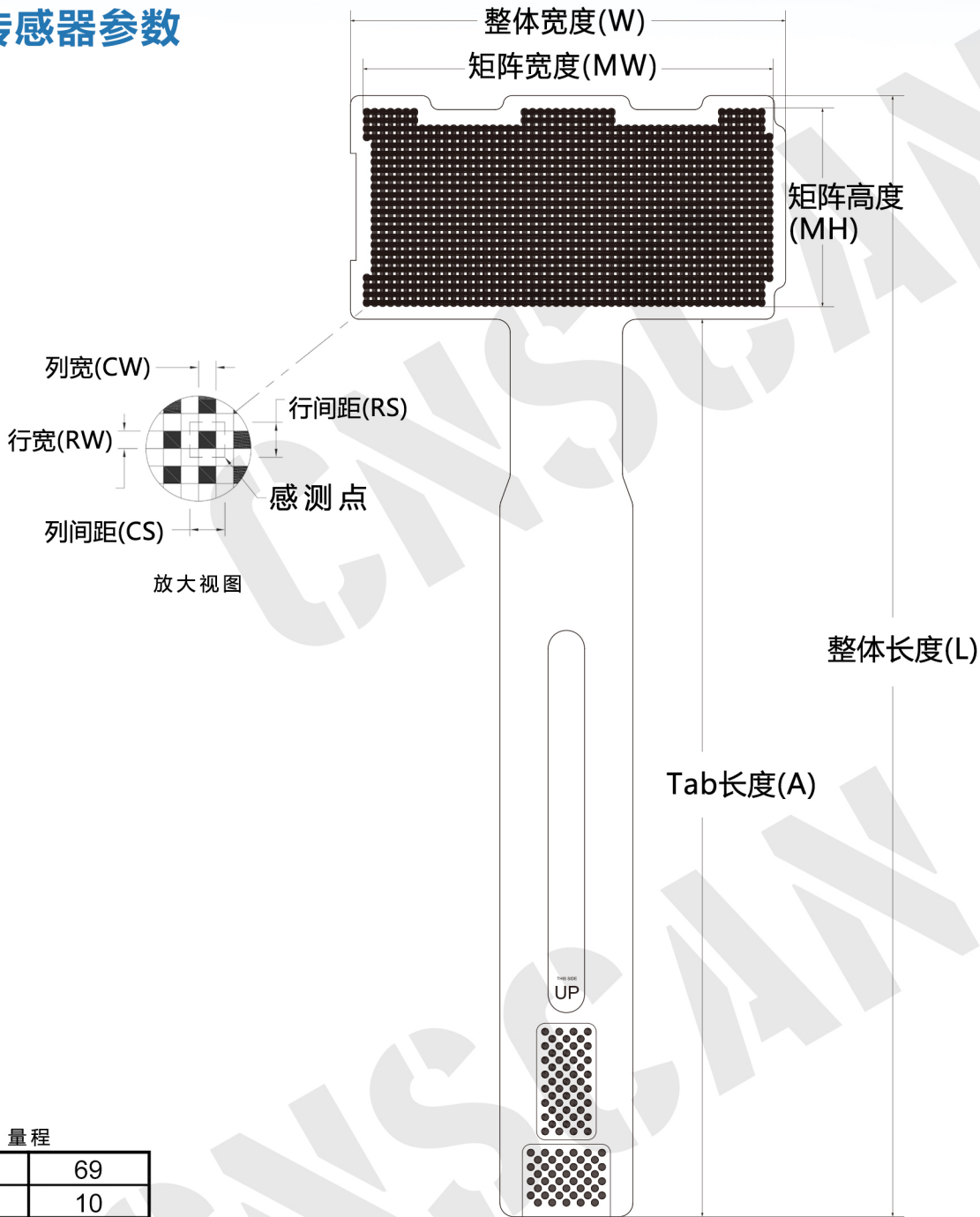
外形尺寸
