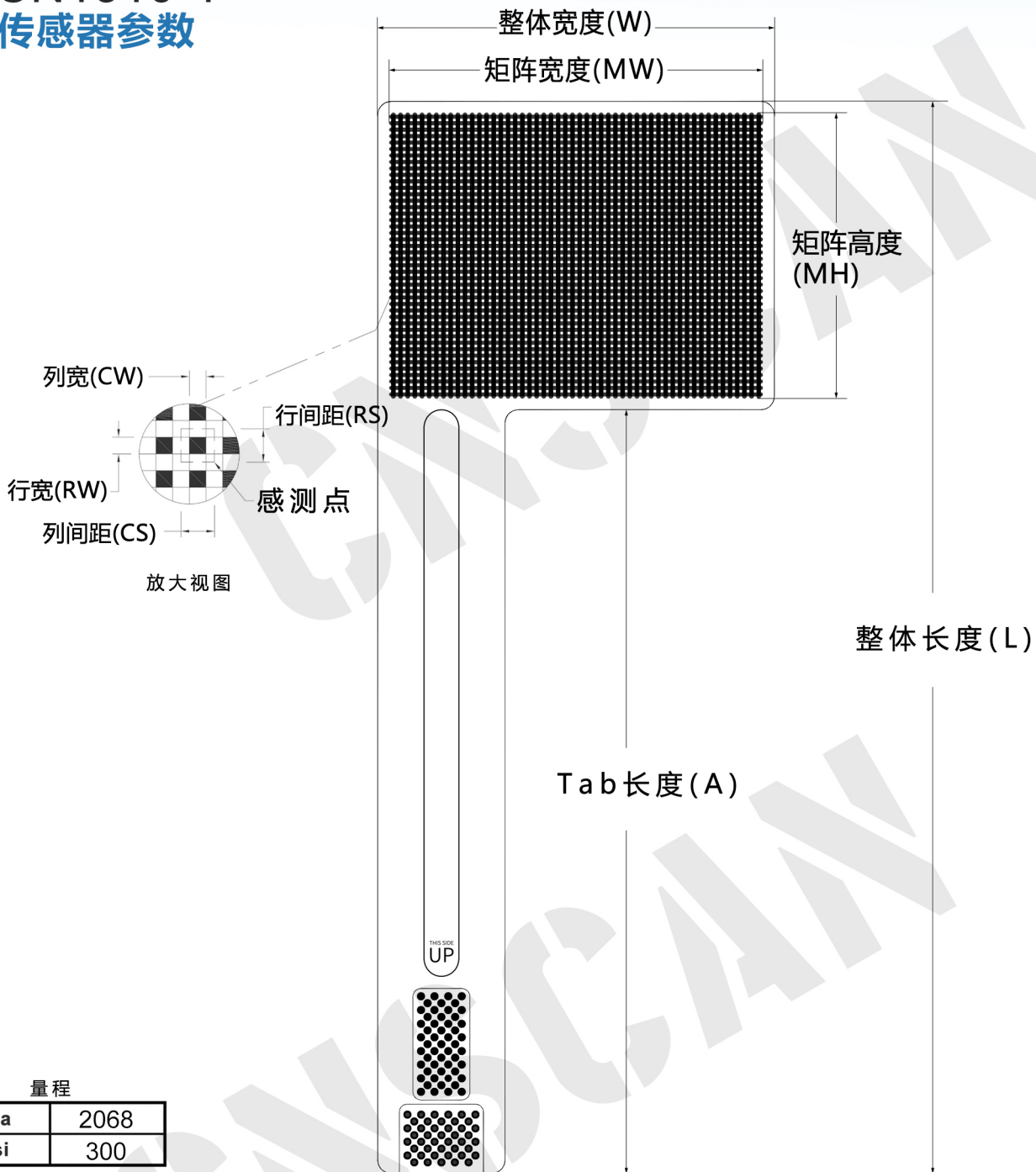
外形尺寸
