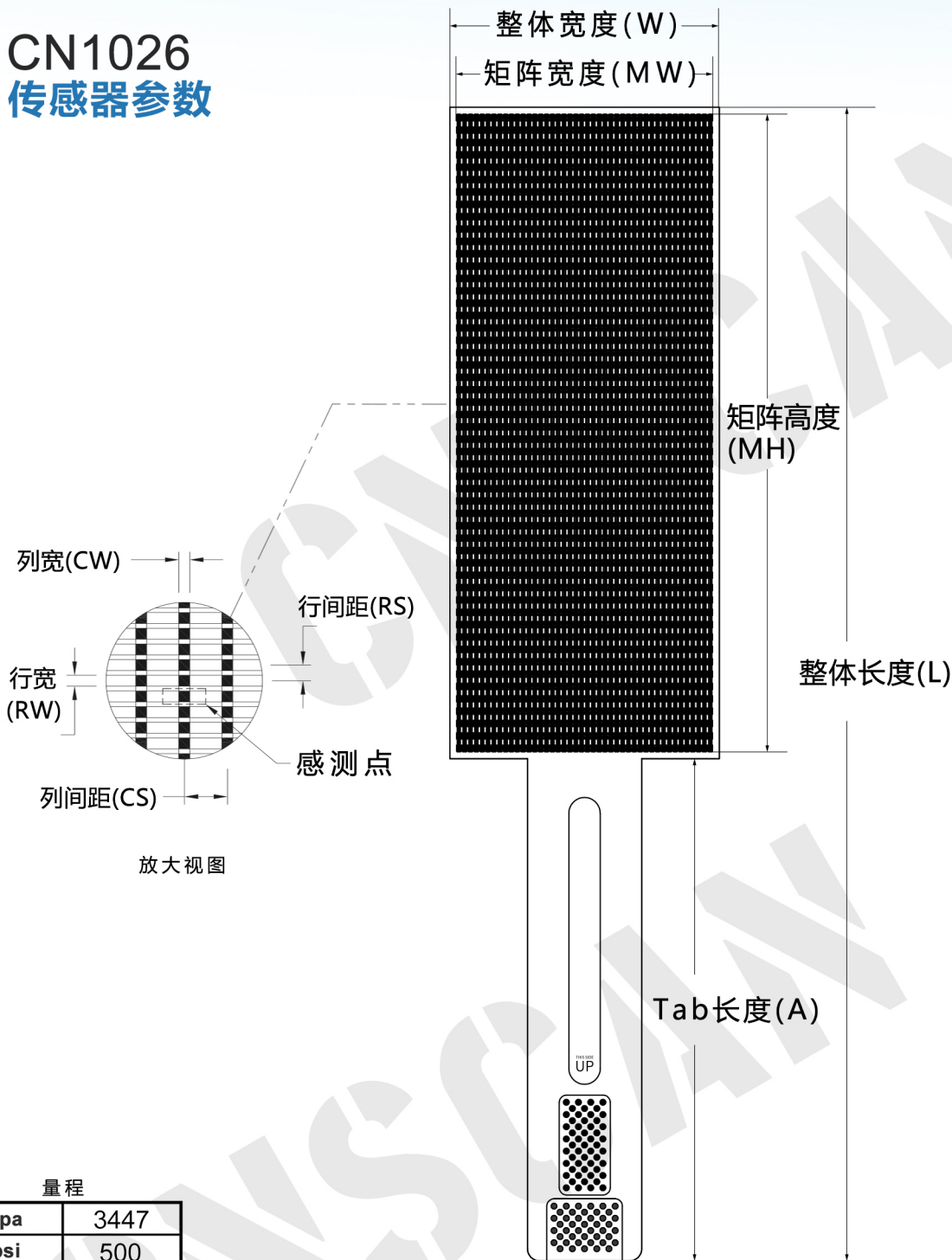
外形尺寸
