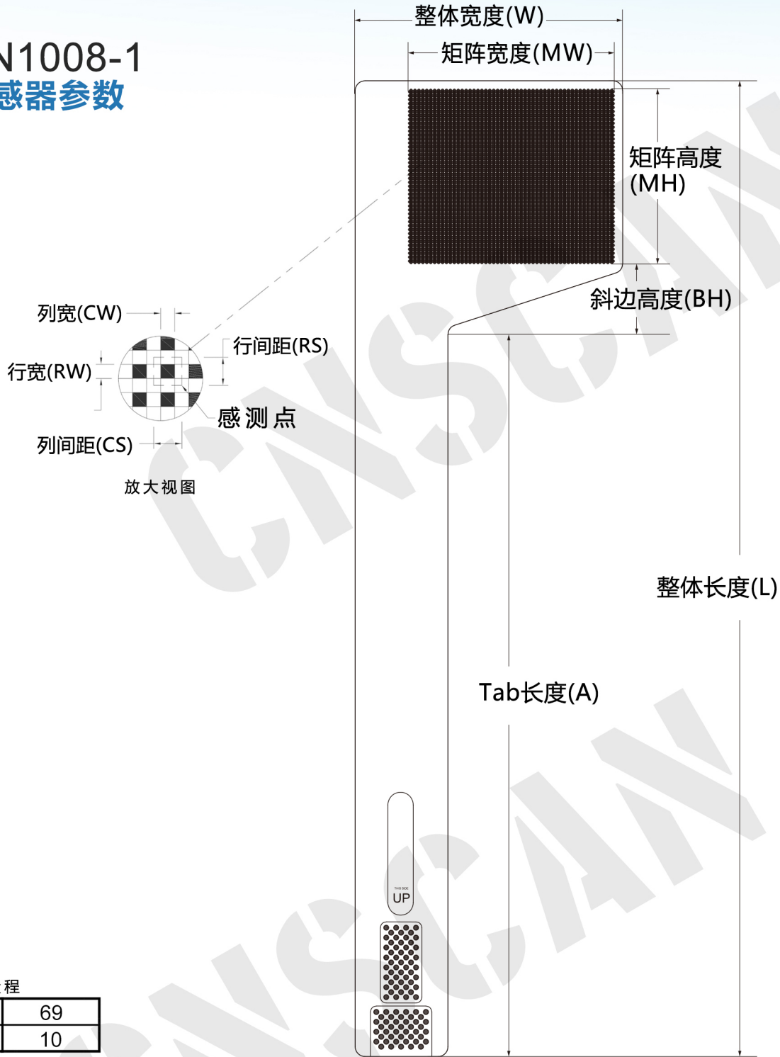
外形尺寸
