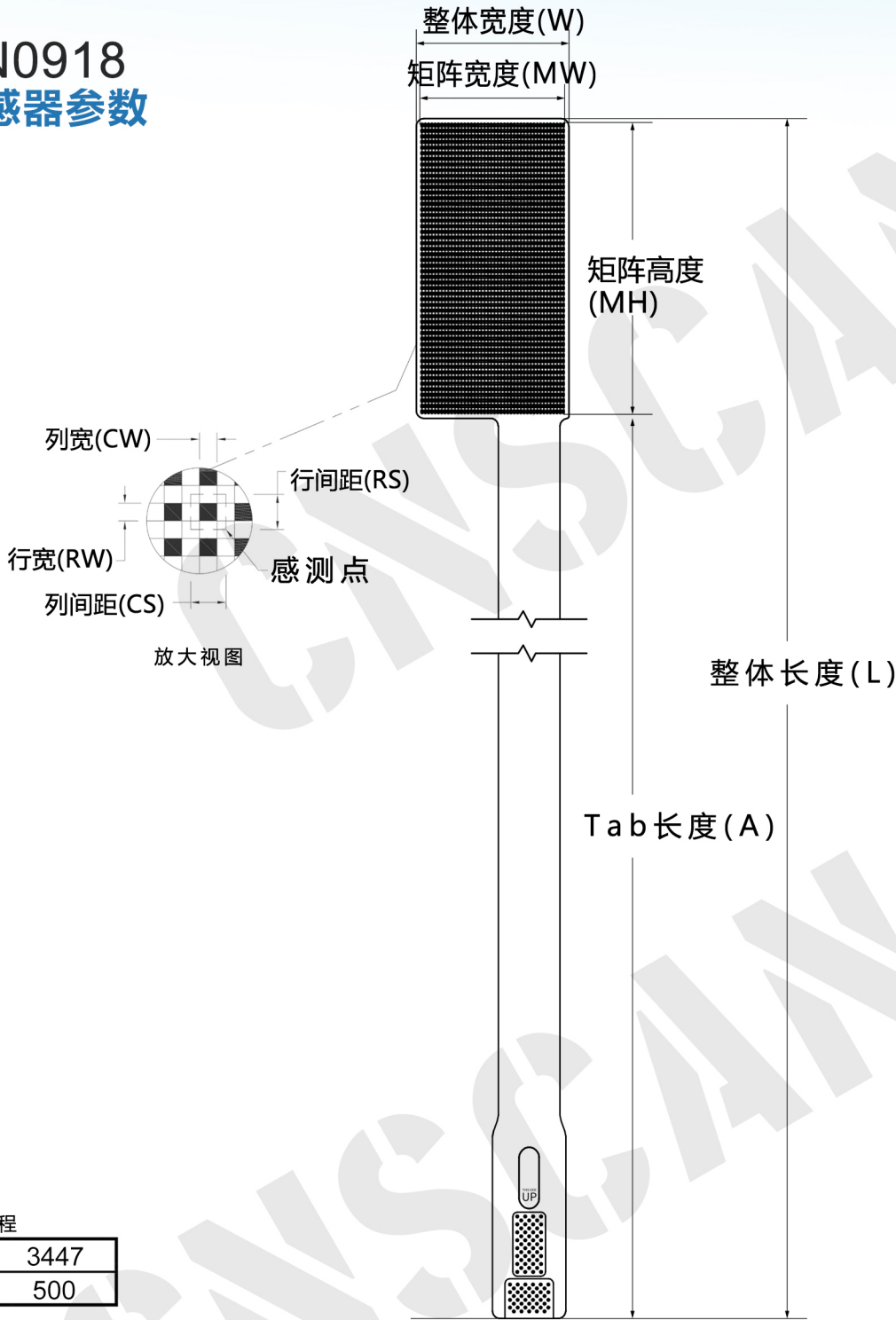
外形尺寸
