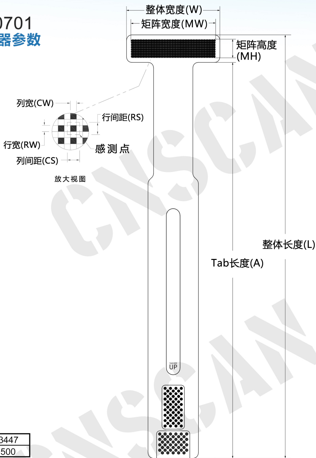
外形尺寸
