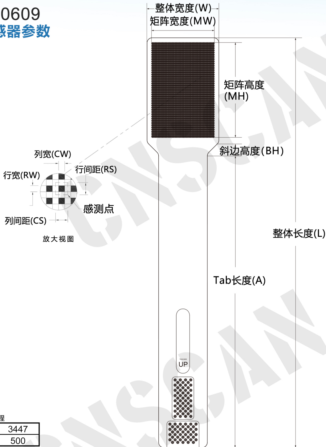
外形尺寸
