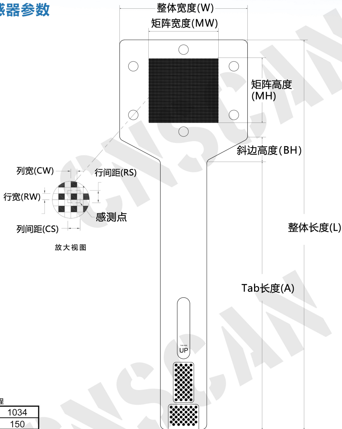
外形尺寸
