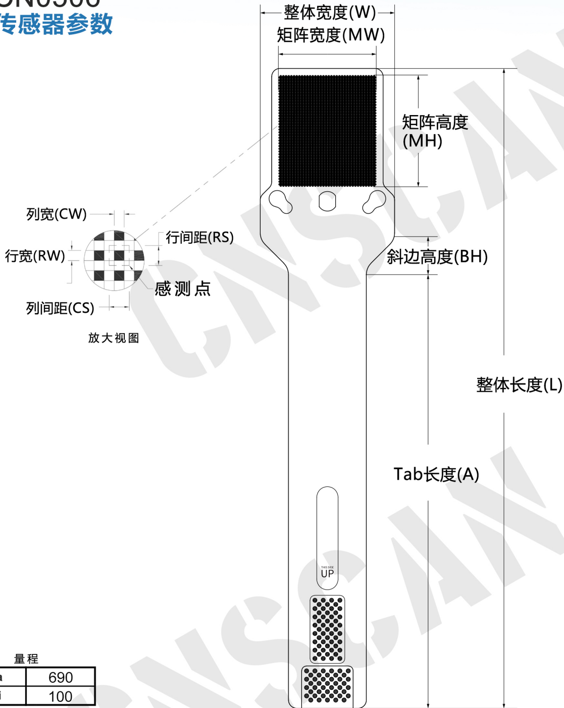
外形尺寸
