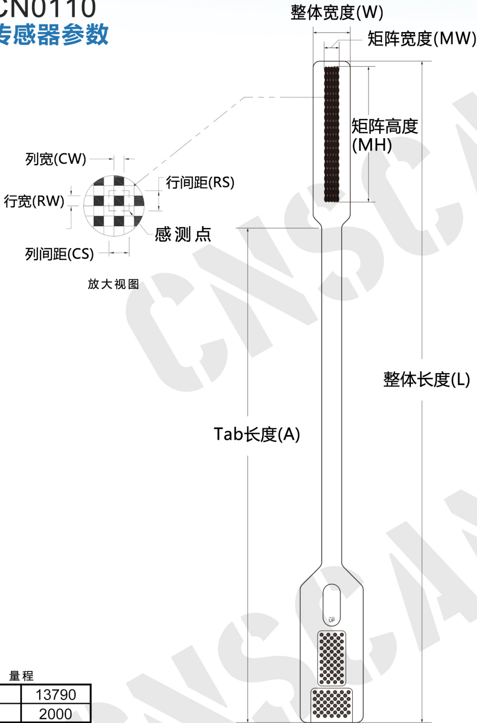
外形尺寸
