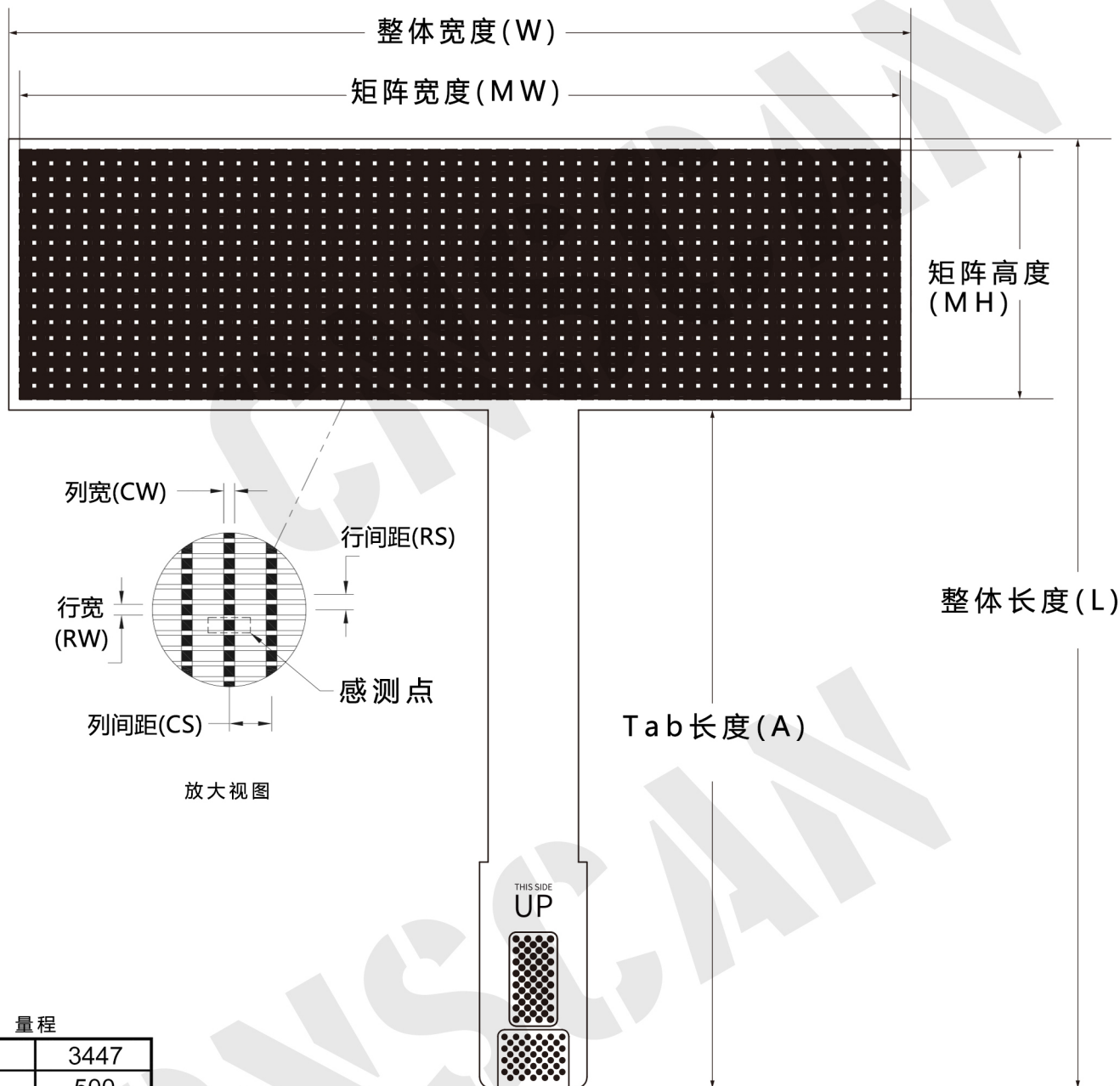
外形尺寸
