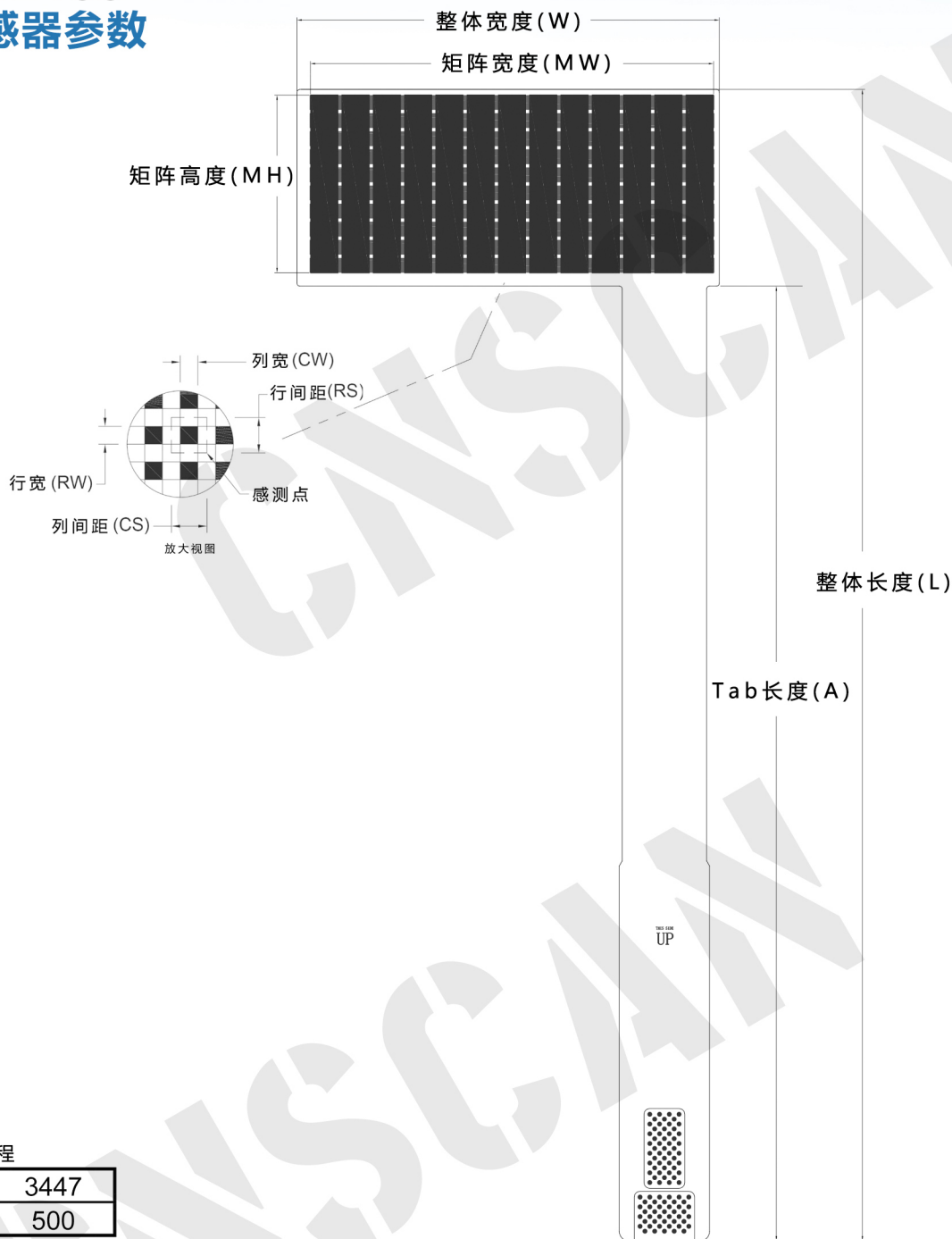
外形尺寸
