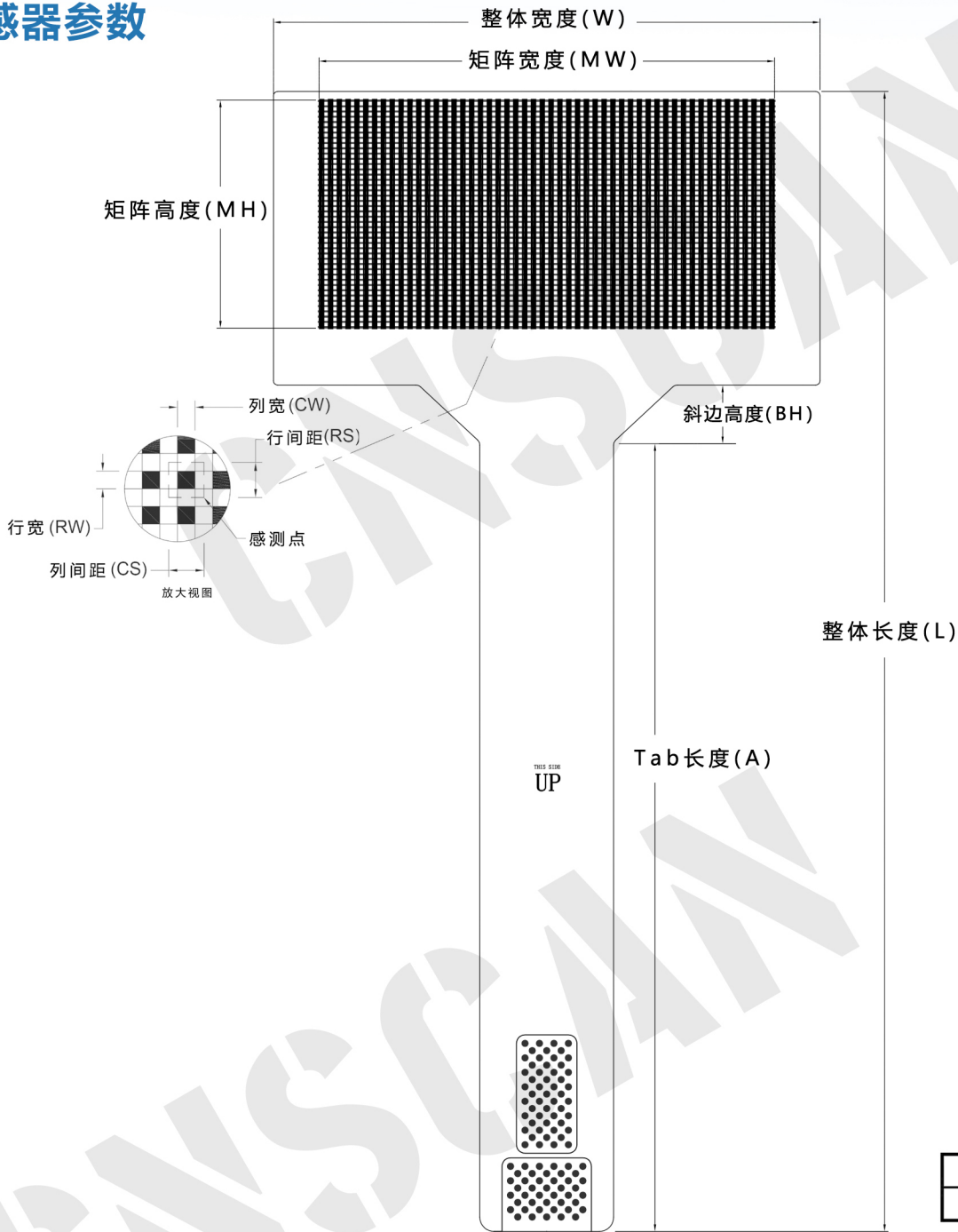
外形尺寸
