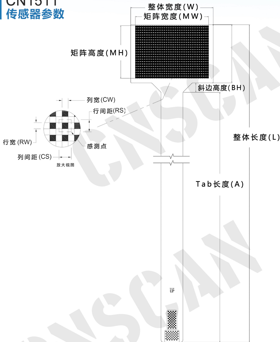
外形尺寸
