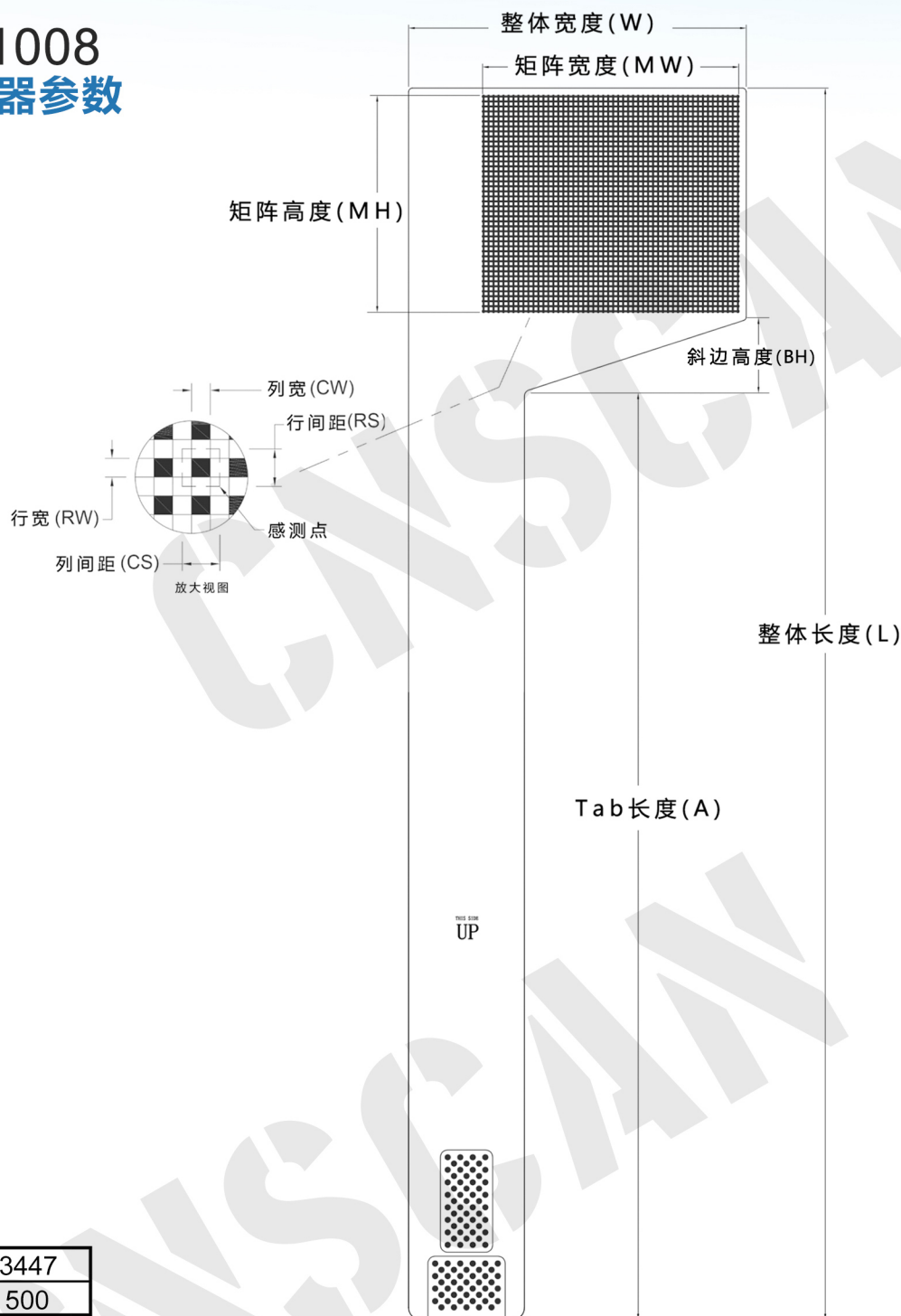
外形尺寸
