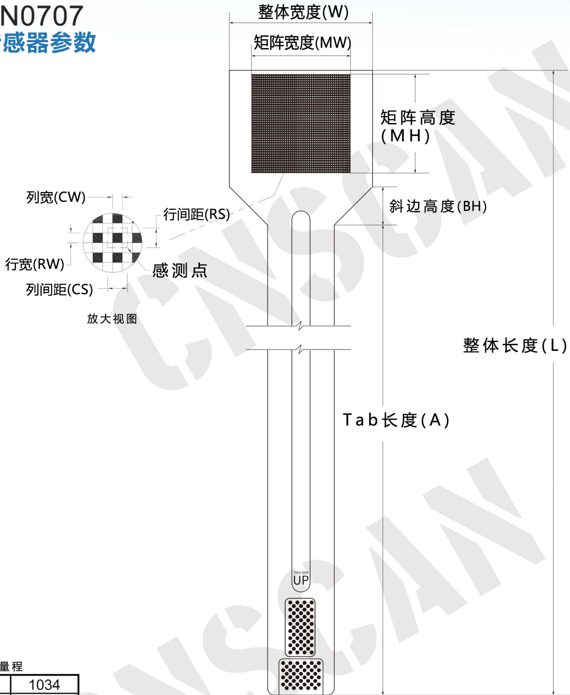
外形尺寸
