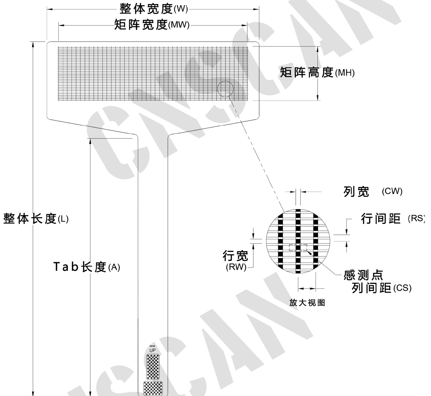
外形尺寸
