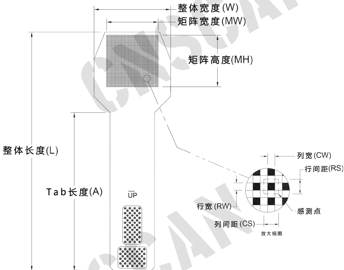
外形尺寸
