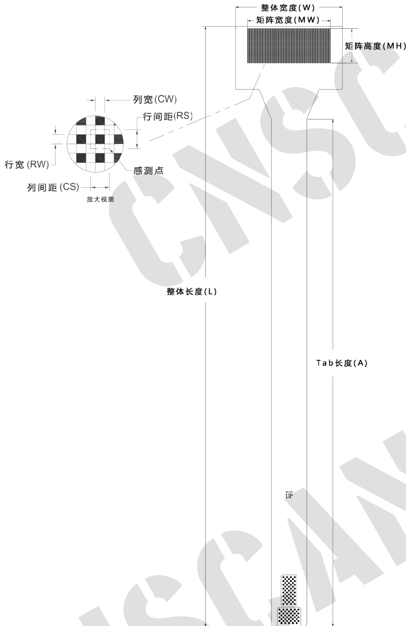
外形尺寸
