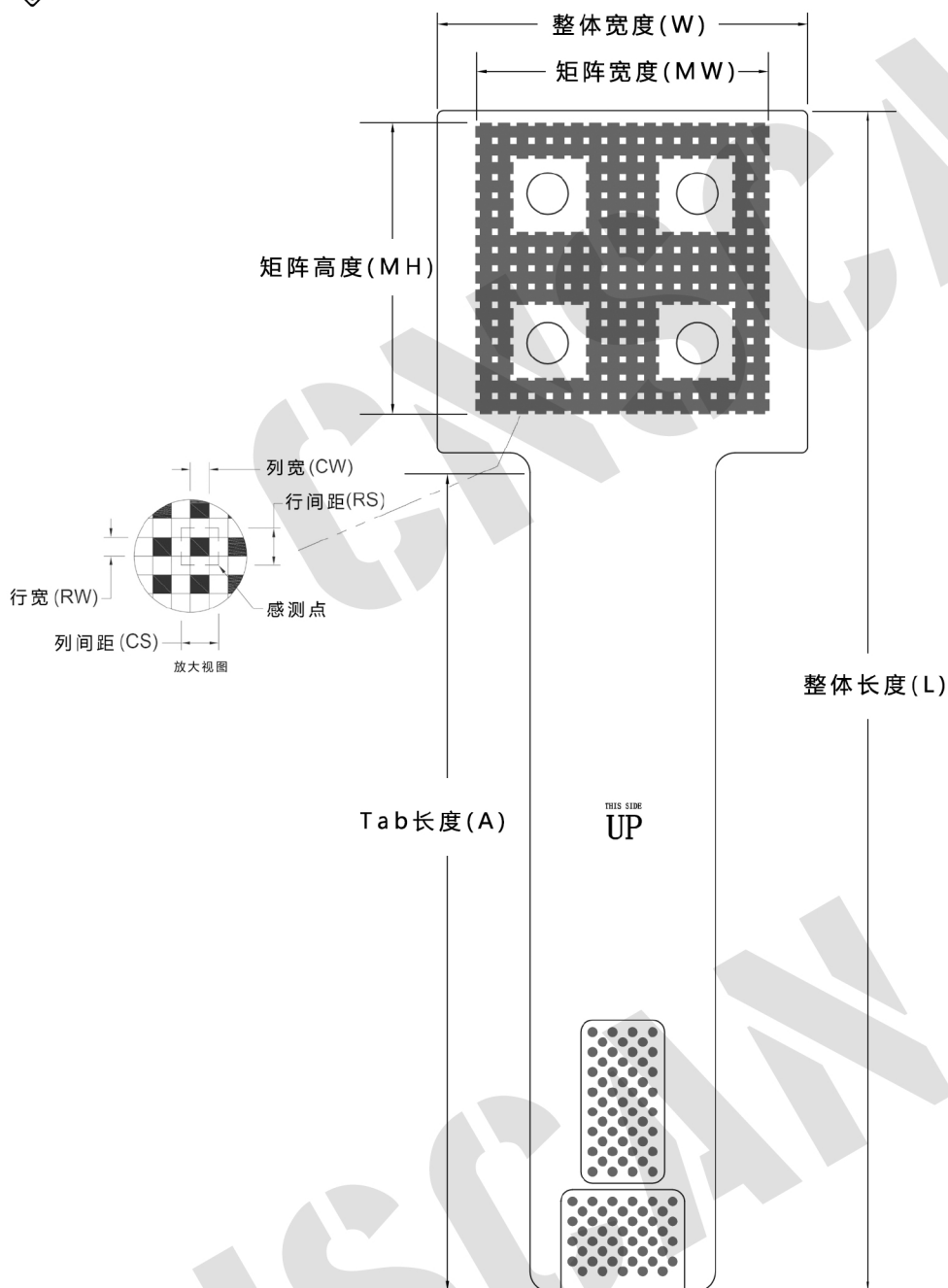
外形尺寸
