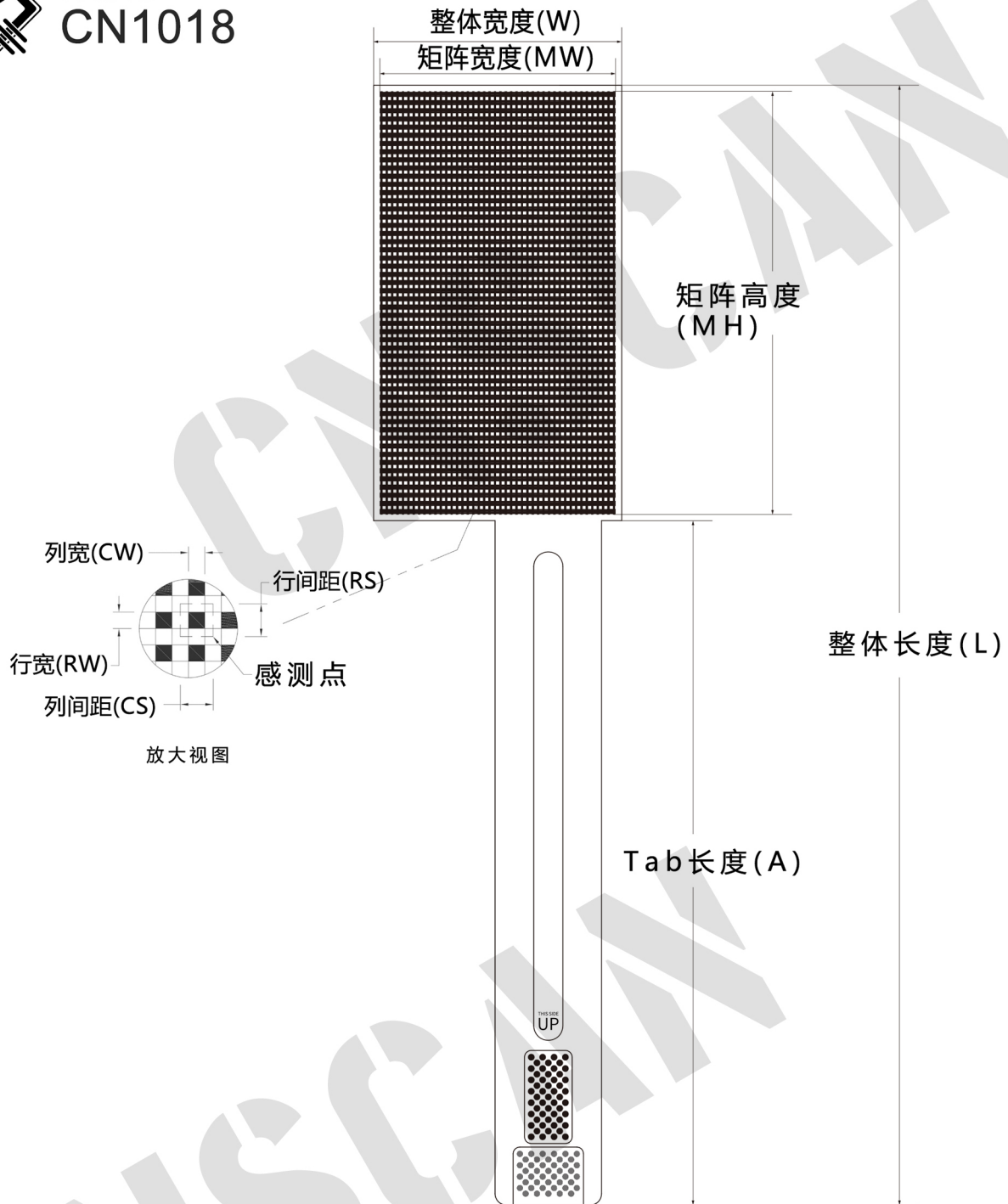
外形尺寸
