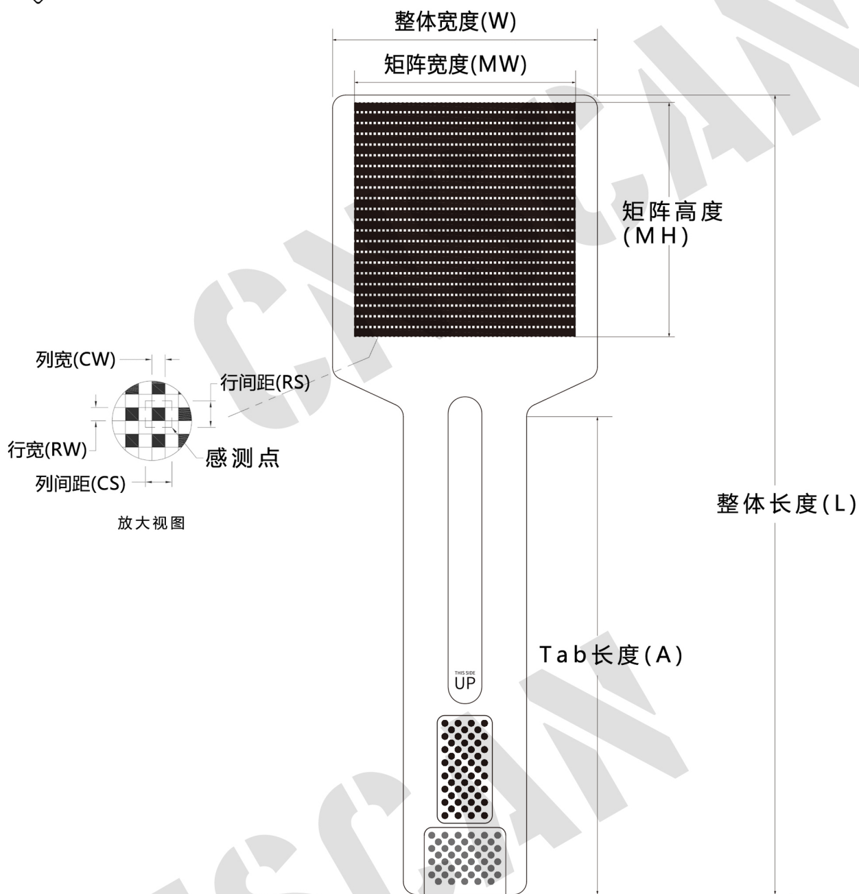
外形尺寸
